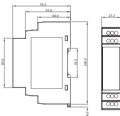
W×H×L=23.2×110.0×70.5(mm)
